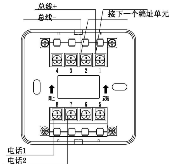
SB8304手动报警按钮接线图
