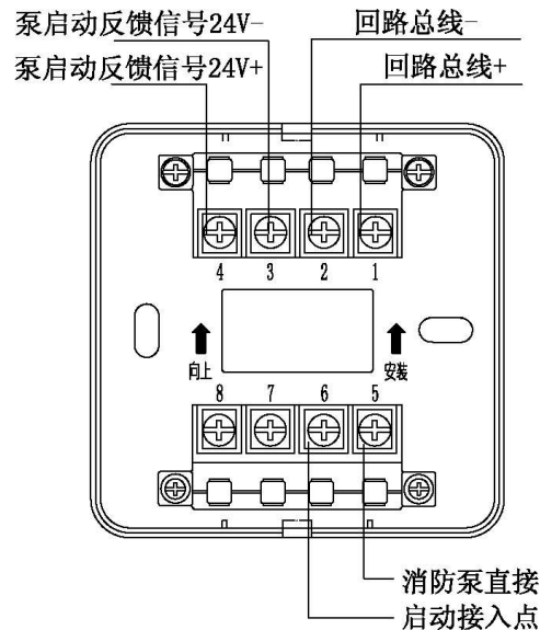
SB8304/H消火栓接线图
